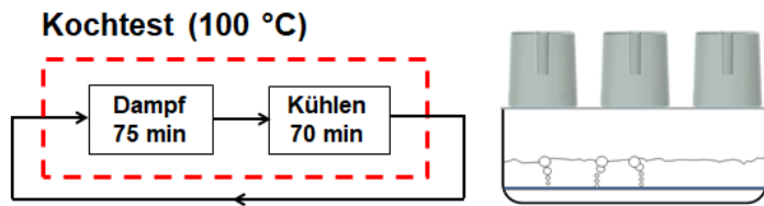
Abbildung: Kochtest Bauteile aus Grilamid TR HT 170 bleiben selbst nach 1'000 Kochzyklen formstabil und transparent.
