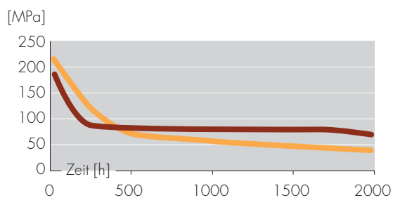
Bruchspannung nach Lagerung in Wasser bei 140°C
